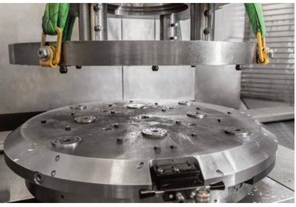
Acht AMF-Nullpunktspannmodule sind in einer Zwischenplatte eingelassen, auf der die Grundplatte für die Werkstückspannung aufsetzt.
