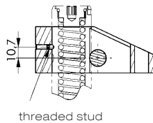
threaded stud
